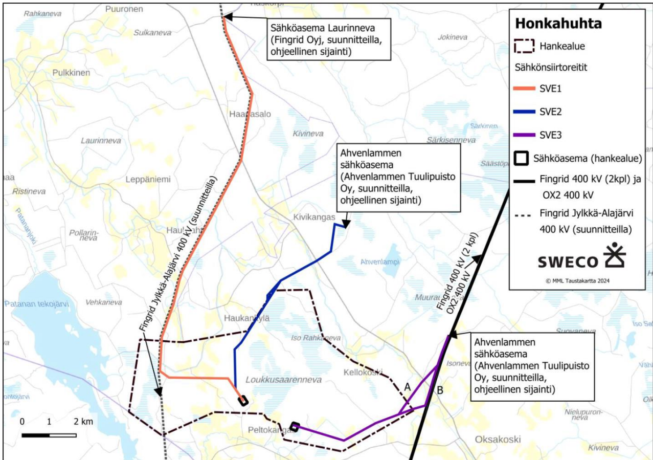
Kuva 2. Hankkeessa suunnitellut sähkösiirron reittivaihtoehdot.
